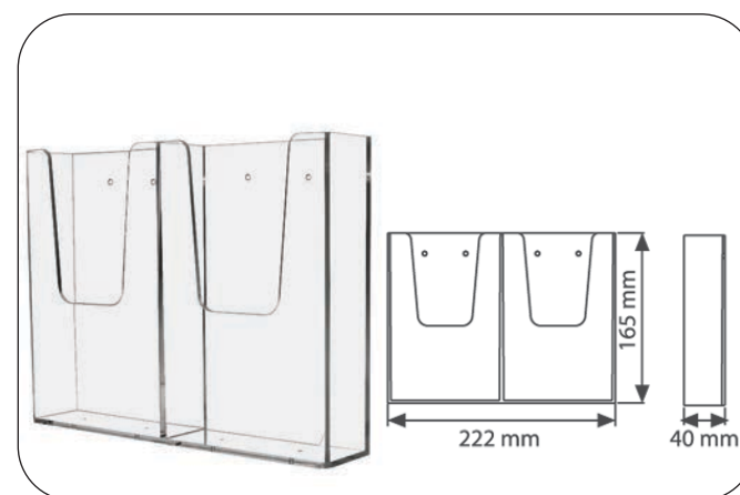
Codice art. Descrizione L.P. MTW110 Portabrochure da parete 2 f.ti 1/3 di A4 cm. 10x21 7
